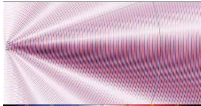
Simulation einer NeodymLine 16 bei 4000 Hz
